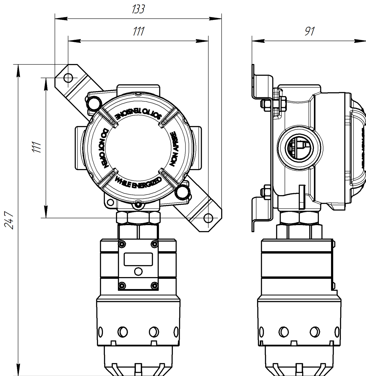
Рисунок Б.4 – Габаритный чертёж газоанализатора с клеммной коробкой
