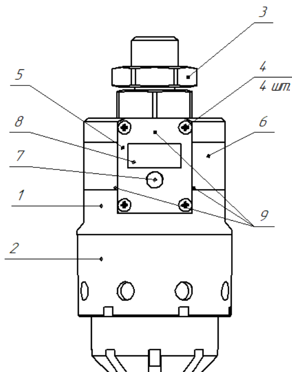
Рисунок 2 – Основные элементы газоанализатора
