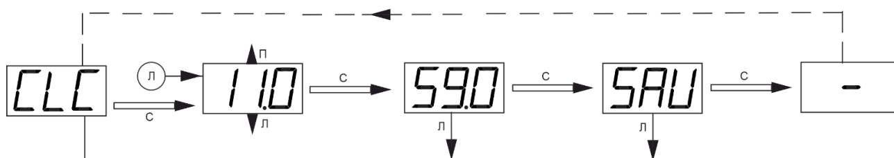
Рисунок 7 – Корректировка диапазона (чувствительности)
