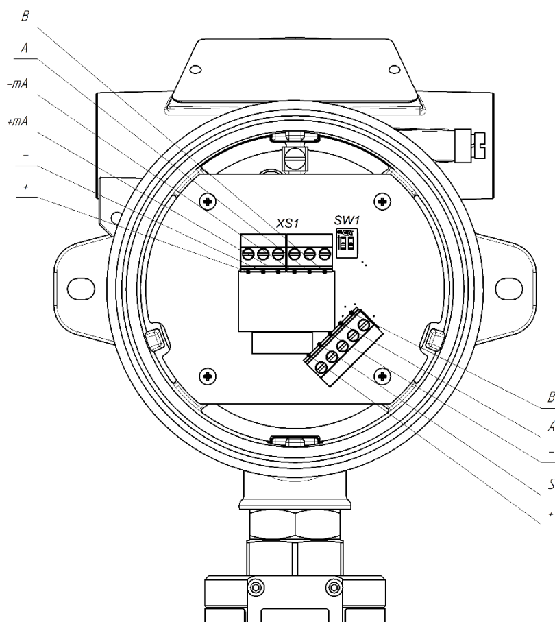
Рисунок 4.1 – Чертеж подключения с опцией переключения режима токовой петли
