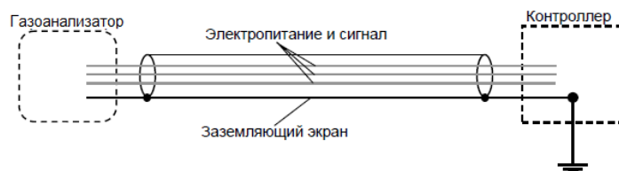
Рисунок 4 – Заземление экранированного кабеля
