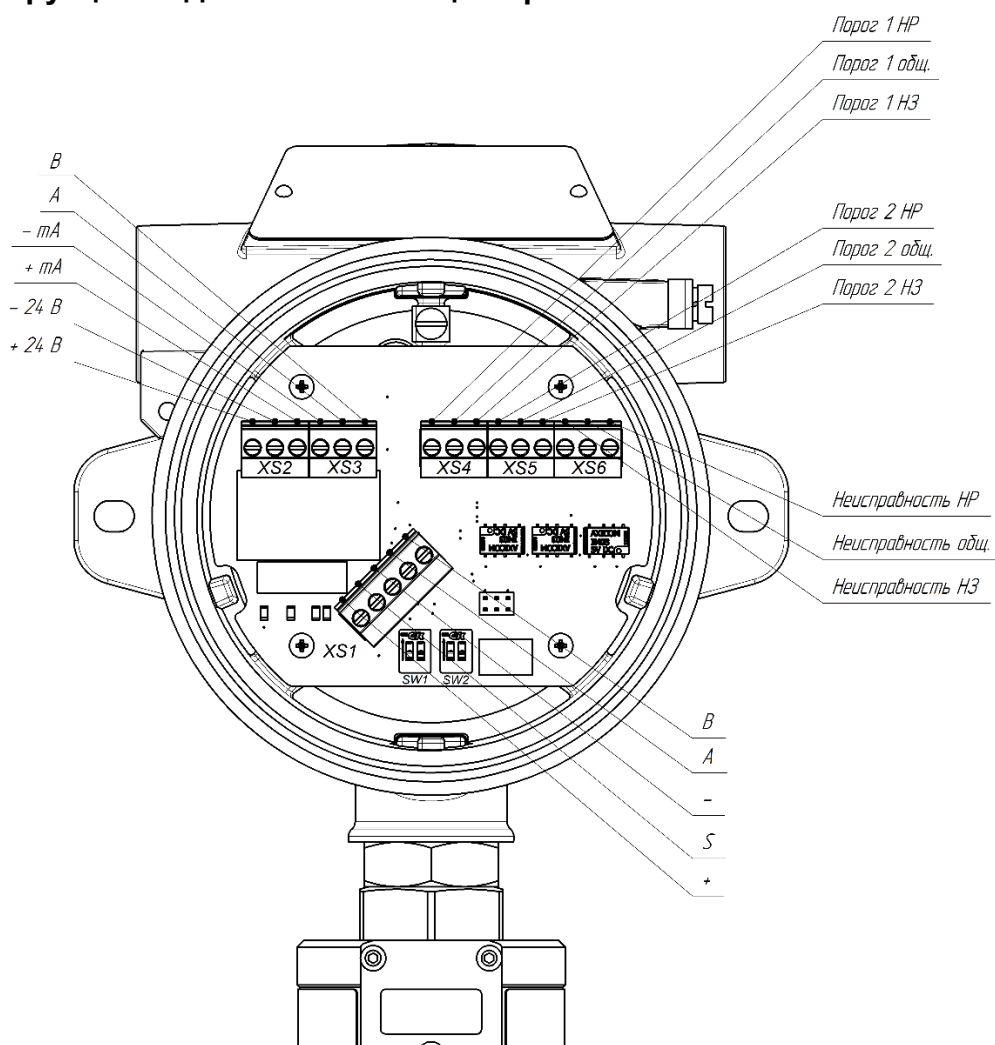
Рисунок 4.2 – Чертеж подключения с опцией переключения режима токовой петли
