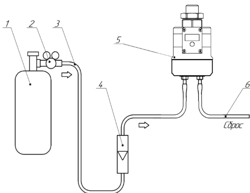
Рисунок 5 – Схема соединений для корректировки газоанализатора
